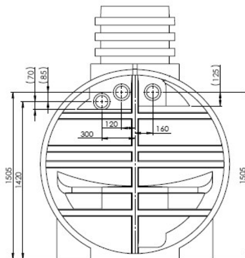
Eco-Line 5000 Litrů
