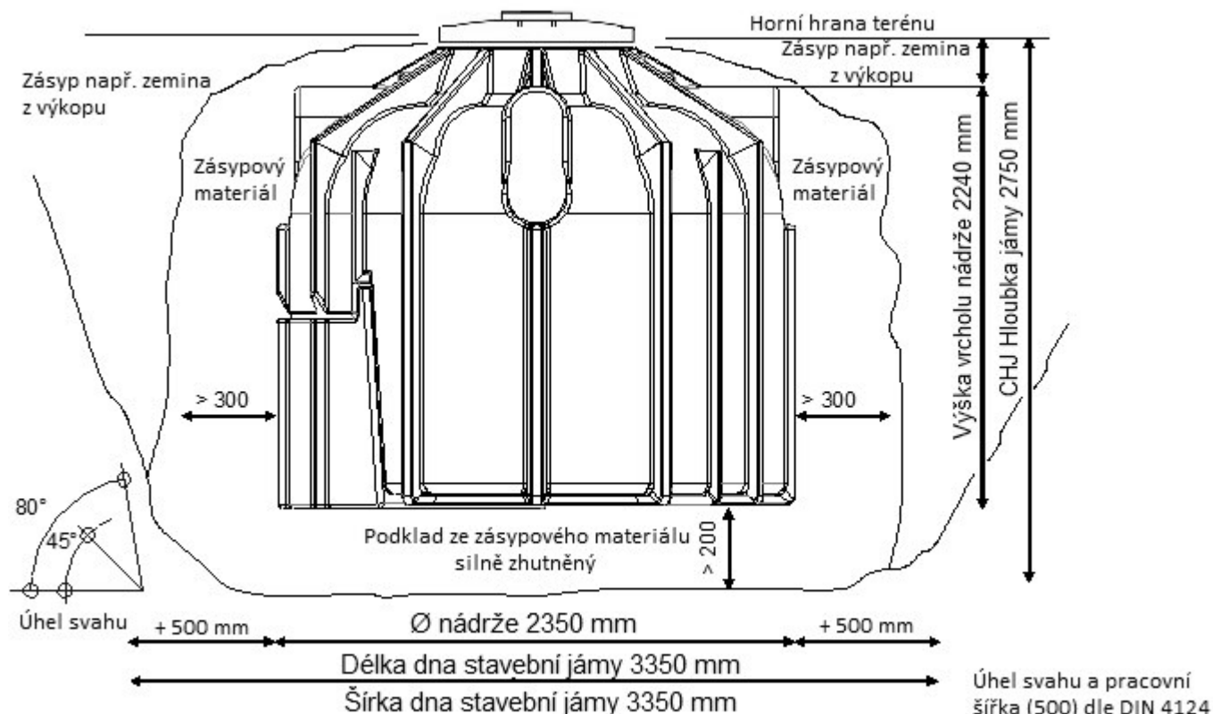
Obr. 2: Montážní velikosti
